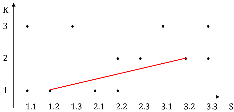
2.6. G(3.2, 1.3)
