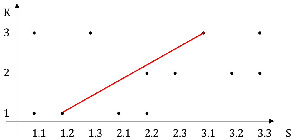
2.3. G(3.1, 1.3)
