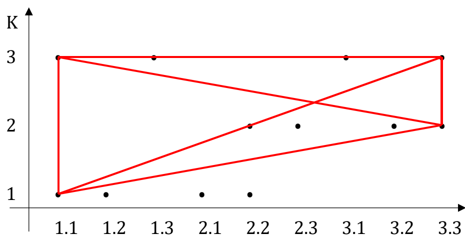
2.7. G(3.3, 1.1)
