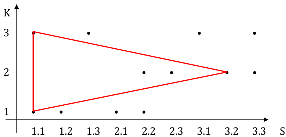
2.4. G(3.2, 1.1)
